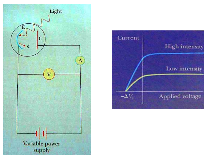
ภาพที่ 18-5 การทดลองโฟโตอิเล็กทริกและกราฟที่ได้จากการทดลอง
